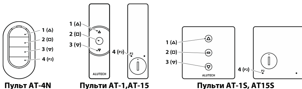
Рисунок 2 – Зовнішній вигляд пультів радіокерування й призначення кнопок: 1 – Кнопка вгору; 2 – Кнопка стоп; 3 – Кнопка вниз; 4 – Кнопка програмування.
